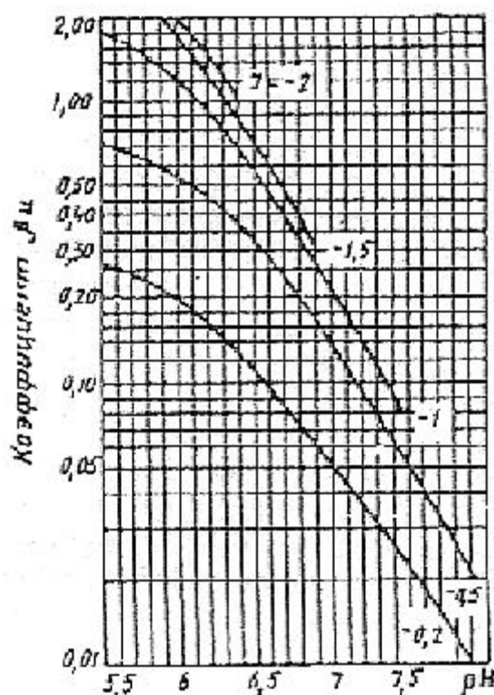
Рис. 4. Номограмма для определения коэффициента b_n при расчете дозы щелочи
