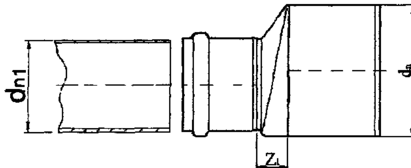
Рисунок 19 – Перехід
