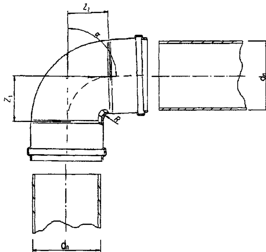
Рисунок 13 – Коліно
