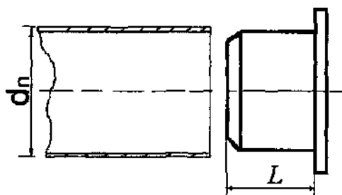
Рисунок 22 – Заглушка
