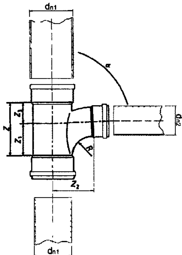
Рисунок 17 – Відгалуження крутозагнуте
