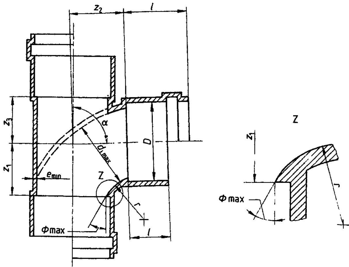
Рисунок Г.6 – Відгалуження крутозагнуте ( 87\frac{1}{2} - 88\frac{1}{2}^\circ )
