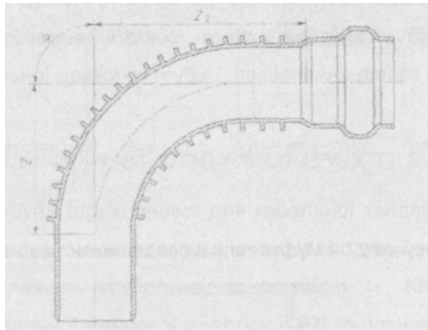
Рисунок 24 – Коліно типу В з внутрішньою манжетою
