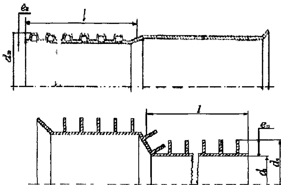
Рисунок 4 – Будівельна довжина труб розтрубних типу В
