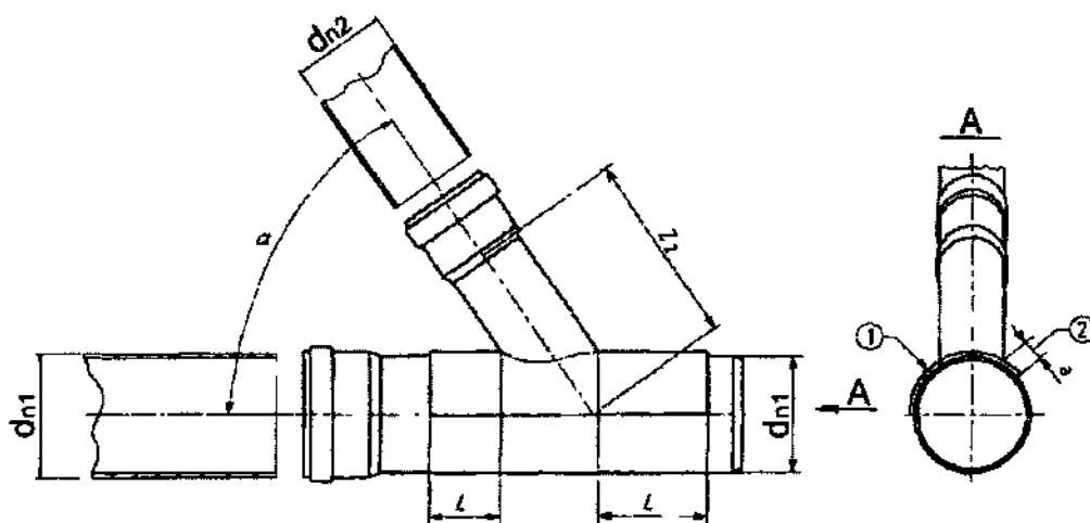
Рисунок 18 – Відгалуження з сідлом
